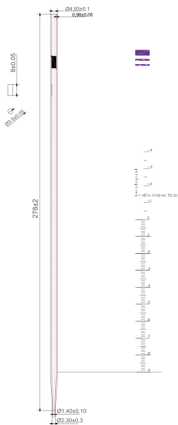
1mL移液管
