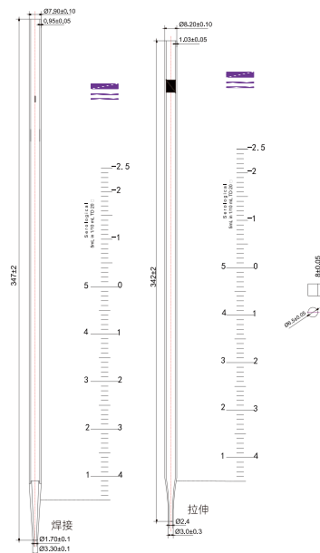
5mL移液管
